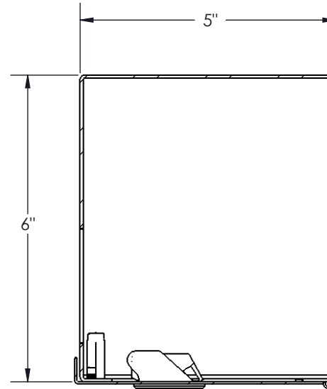
SECTION D-D SCALE 3 : 8
