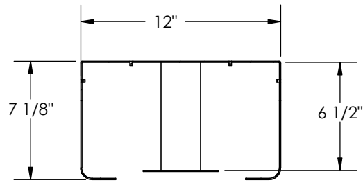
SECTION B-B SCALE 1 : 8
