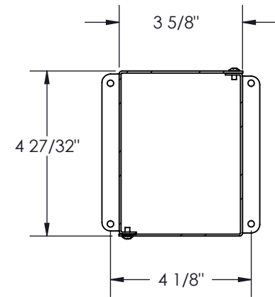
SECTION A-A SCALE 1 : 4
